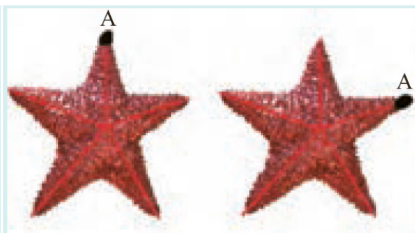
تقارن‌های دورانی
