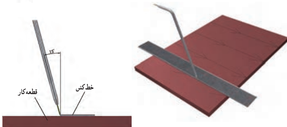
شکل ۱-۴ - روش صحیح خط‌کشی با خط‌کش و سوزن خط‌کش
